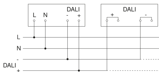
aansluitschema voor DALI-2 APC met DALI-2 IPD
